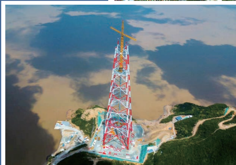
《双平臂落地抱杆》标准填补国内该类产品标准空白，特大跨越输电铁塔组立专用设备列为浙江省装备制造业重点领域首台（套）产品。
